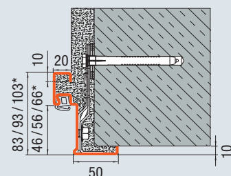
Eckzarge mit Dübelmontage in der Leibung (Mauerwerk / Beton)
