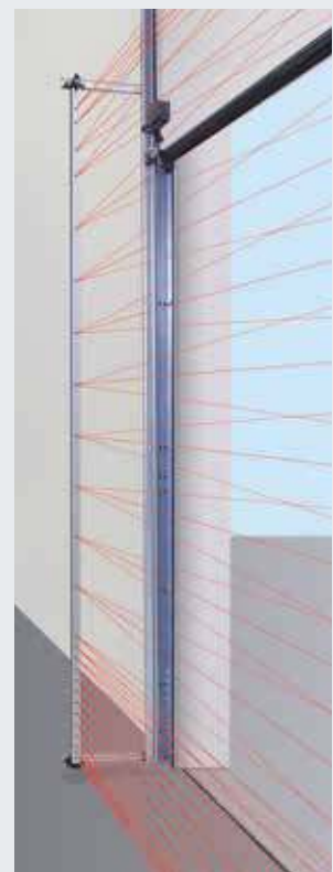
Lichtgitter HLG-V Montage an der Torzarge
